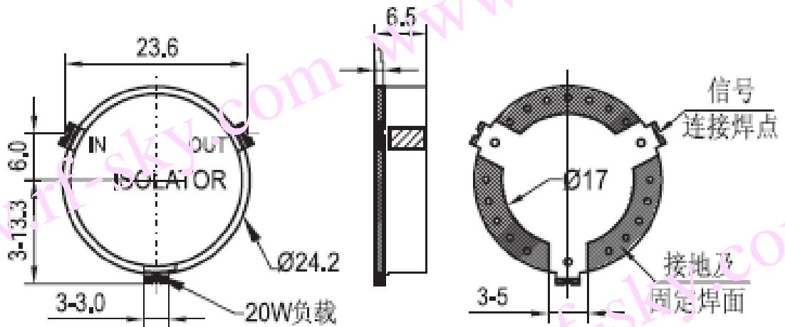
SI070A 安装图
