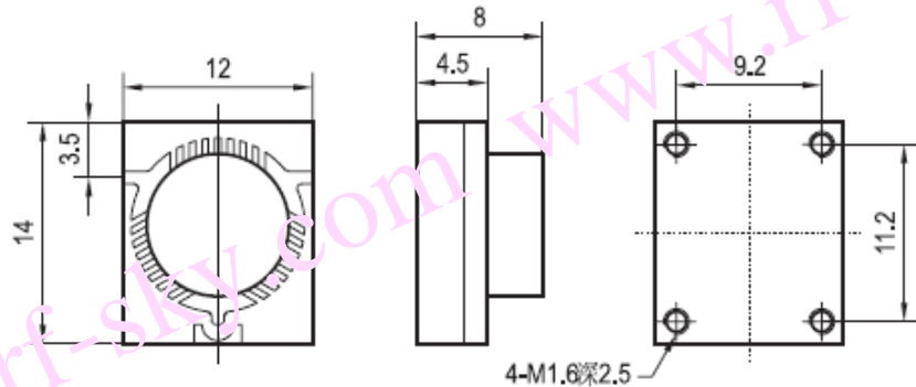
MI400A 安装图
