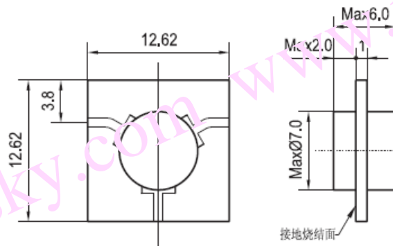
MC550A 安装图
