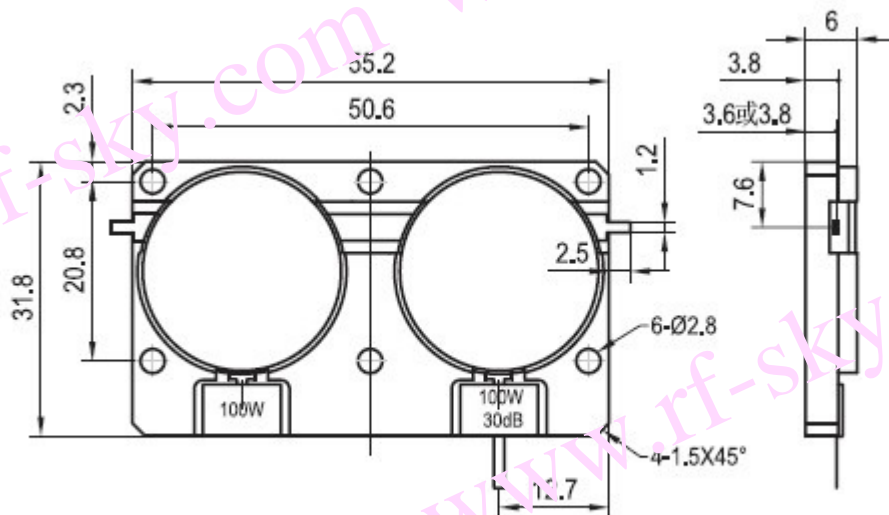
DI970TA-D 安装图
