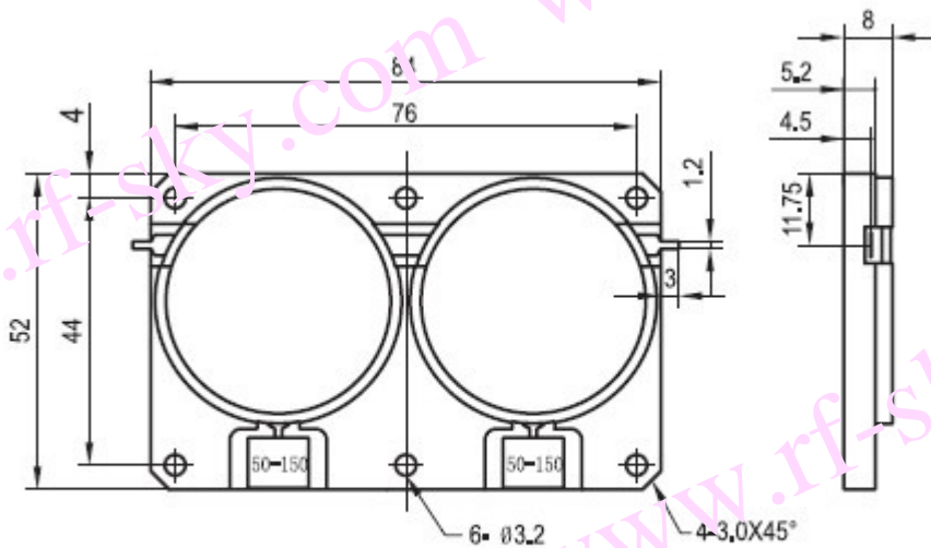
DI030TA-D 安装图
