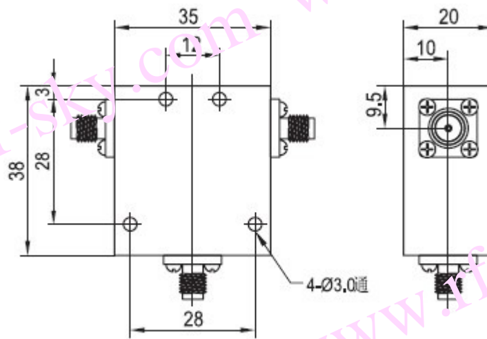
CC040PA 安装图
