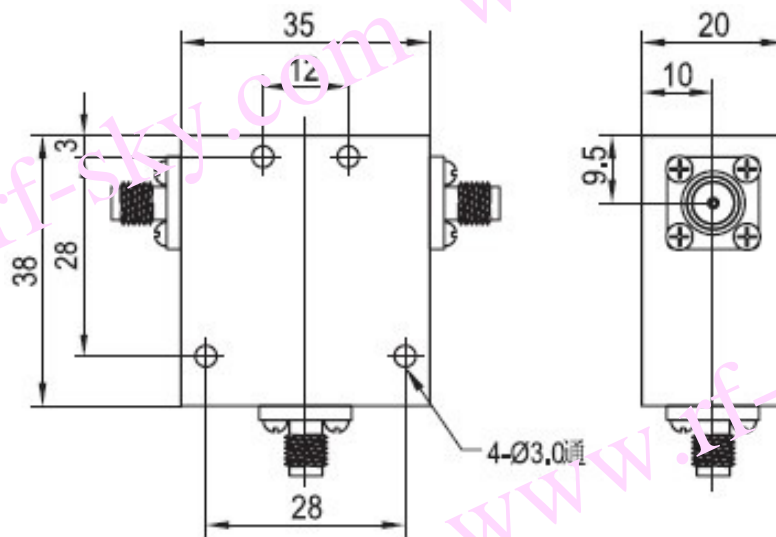
CC040PA 安装图
