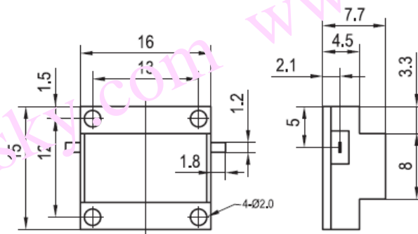
DI900PA-D 安装图
