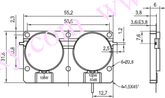
DI070TA-D 安装图
