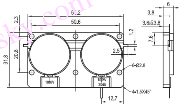
DI070TA-D 安装图
