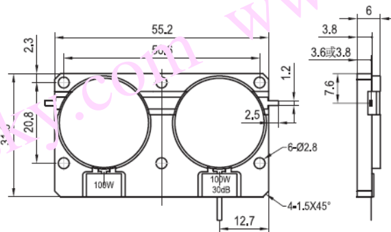
DI070TA-D 安装图
