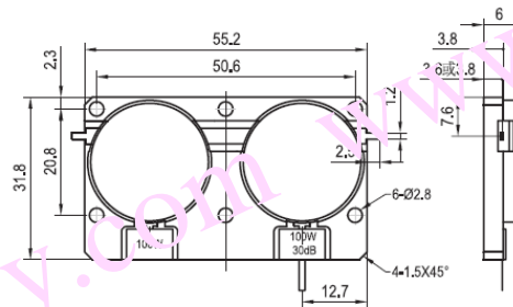
DI070TA-D 安装图
