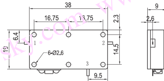
DC170PA-D 安装图
