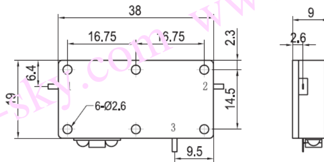
DC170PA-D 安装图
