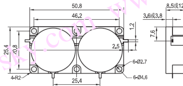
DC070SA-D 安装图
