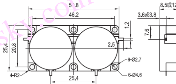
DC070SA-D 安装图
