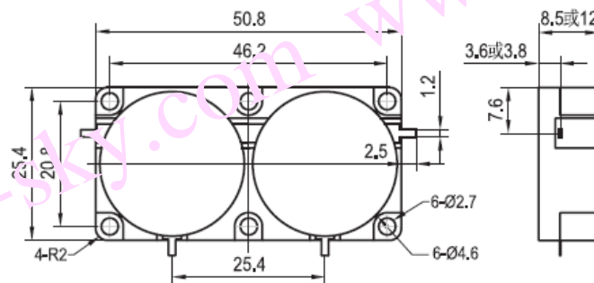
DC070SA-D 安装图
