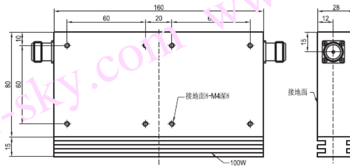
CI003PA-D 安装图
