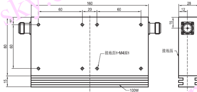
CI003PA-D 安装图
