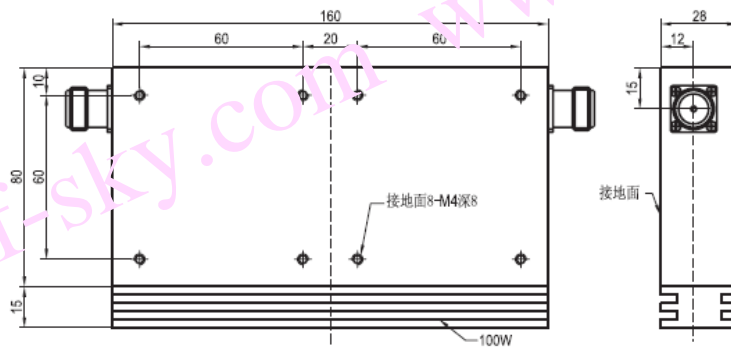
CI003PA-D 安装图
