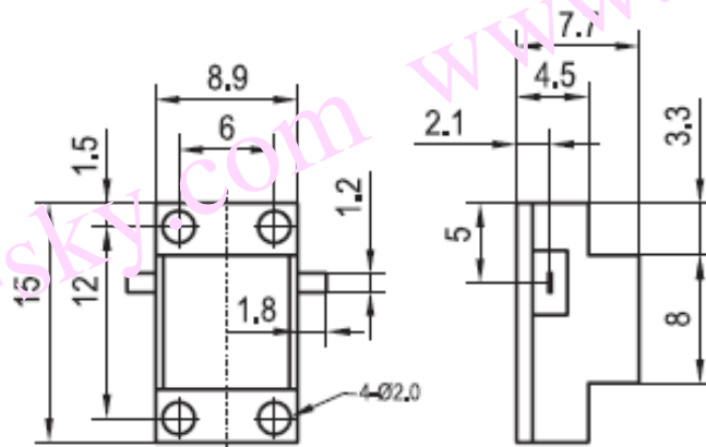
DI800PA 安装图
