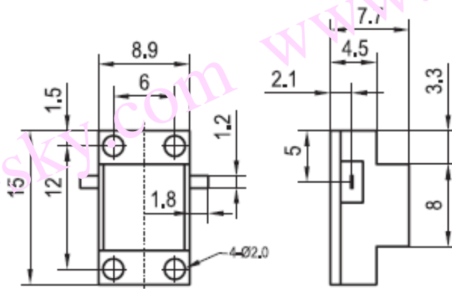
DI800PA 安装图
