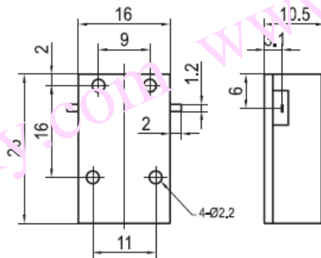
DI350PA 安装图
