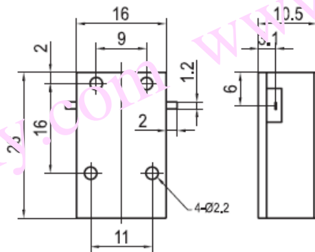
DI350PA 安装图
