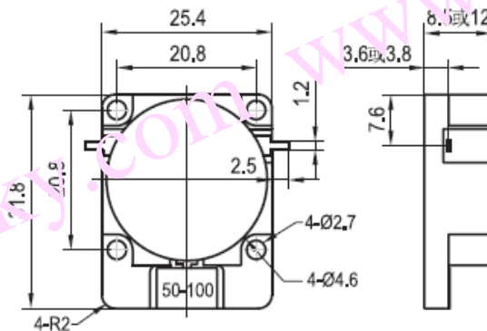
DI070SA 安装图
