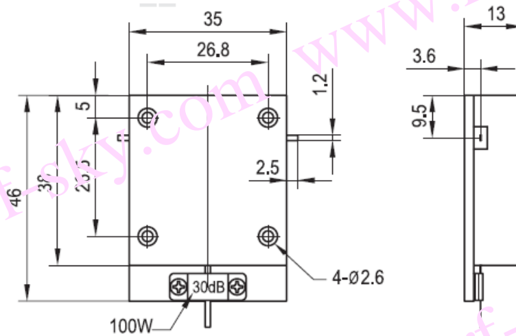
DI040PA 安装图
