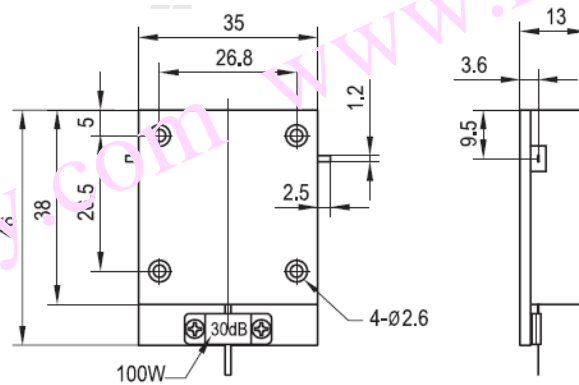
DI040PA 安装图
