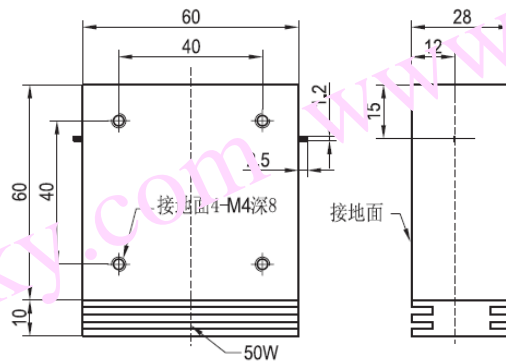
DI007PA 安装图
