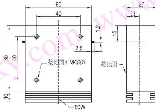
DI007PA 安装图
