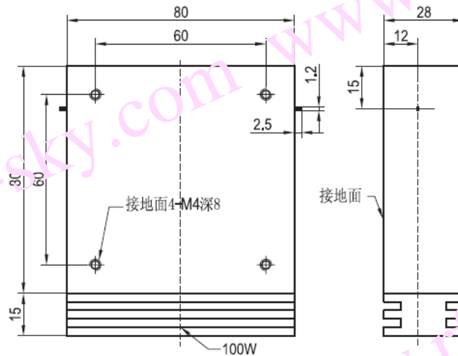
DI003PA 安装图
