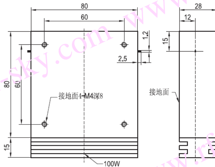
DI003PA 安装图
