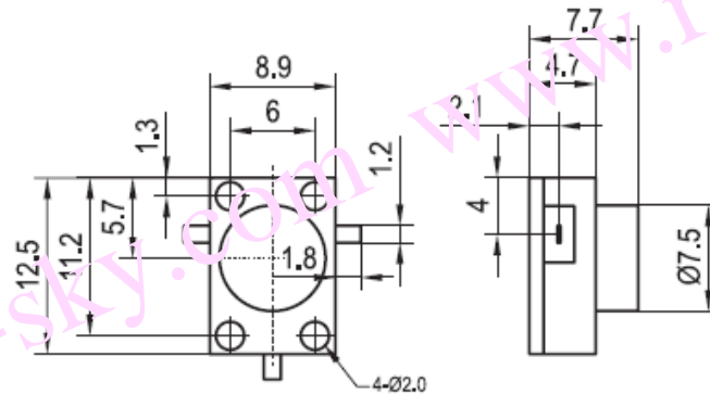
DC800PA 安装图
