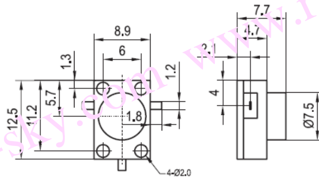
DC800PA 安装图
