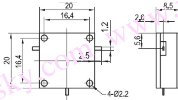
DC080PA 安装图
