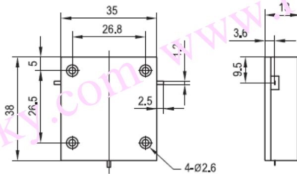
DC040PA 安装图
