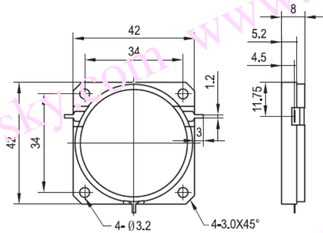
DC030TA 安装图
