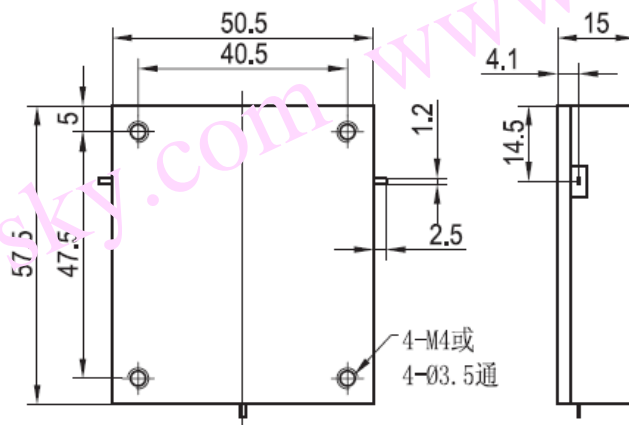
DC020PA 安装图
