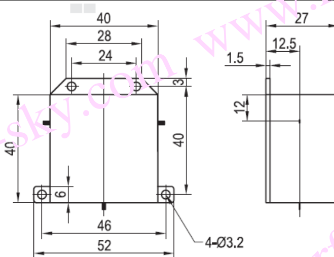
DC010PA 安装图
