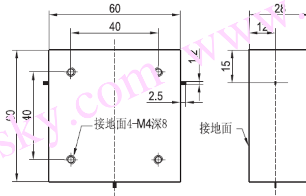
DC007PA 安装图
