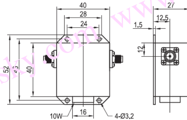
CI010PA 安装图
