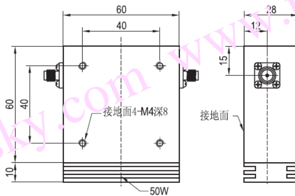
CI007PA 安装图
