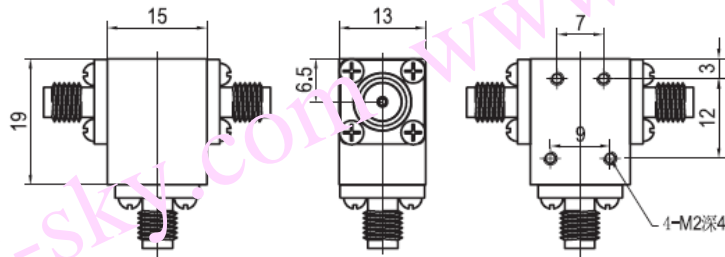
CC650PA 安装图
