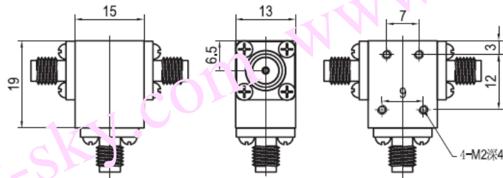
CC650PA 安装图
