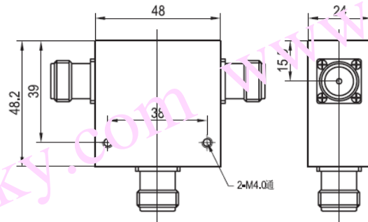
CC030PA 安装图
