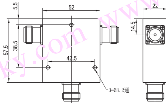
CC020PA 安装图
