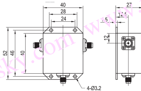
CC010PA 安装图
