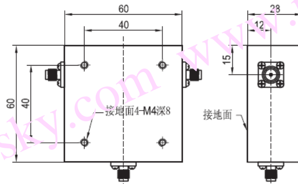
CC007PA 安装图
