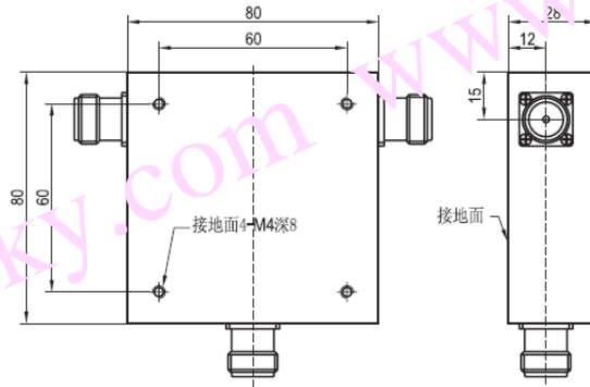
CC003PA 安装图
